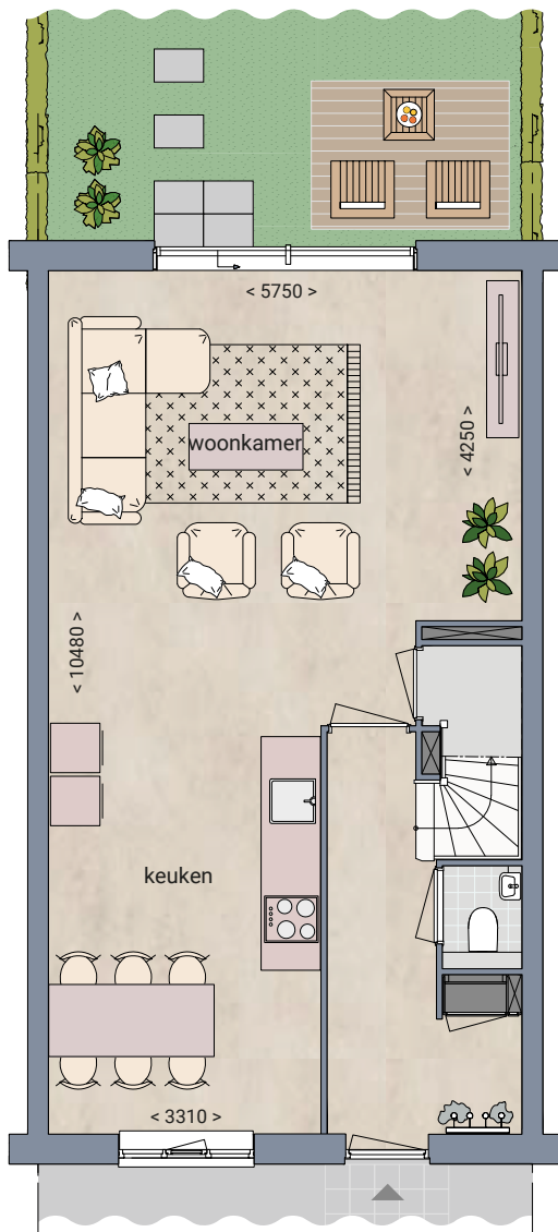
begane grond
