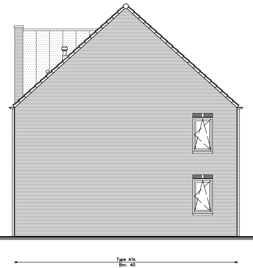
Rechter zijgevel
