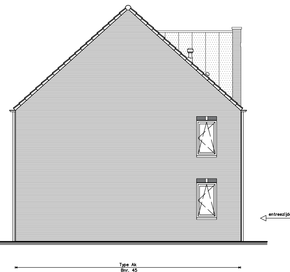
Linker zijgevel
