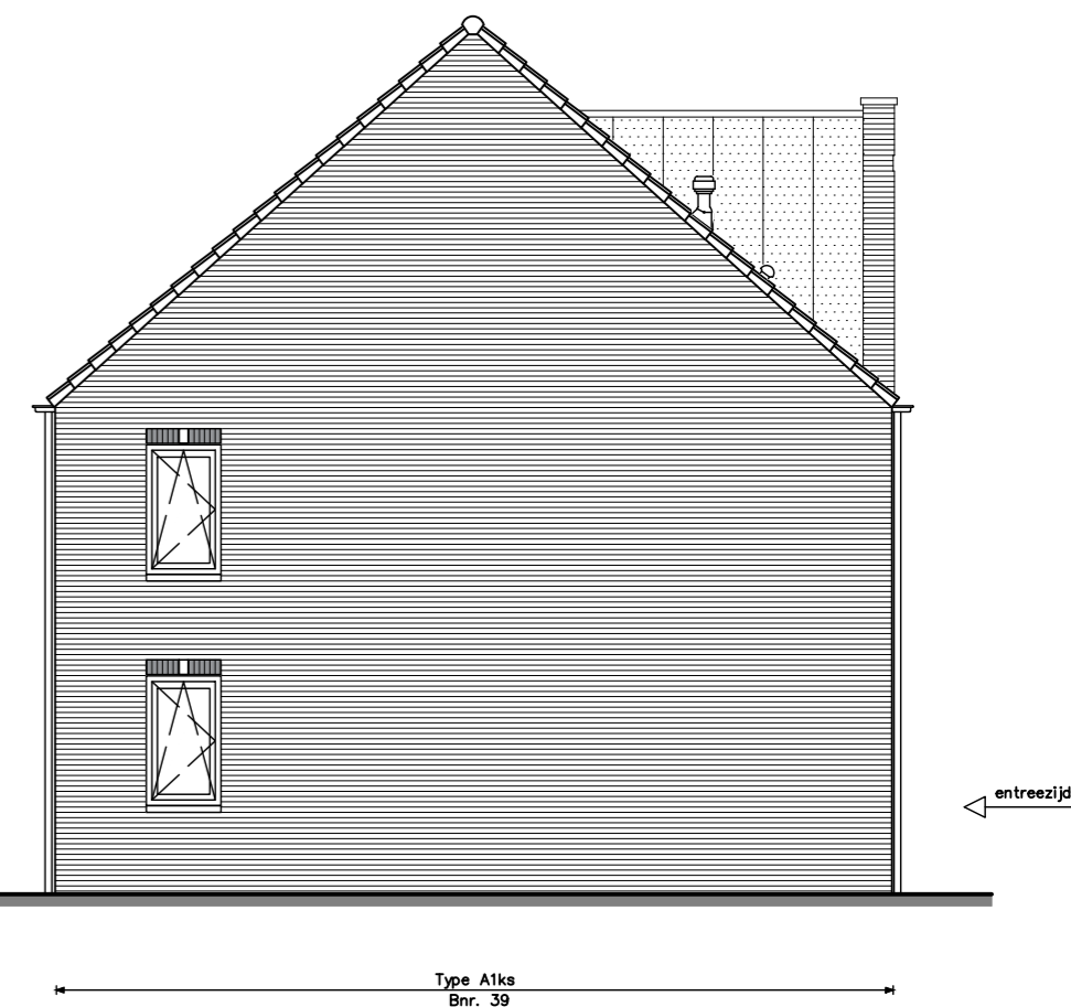
Linker zijgevel
